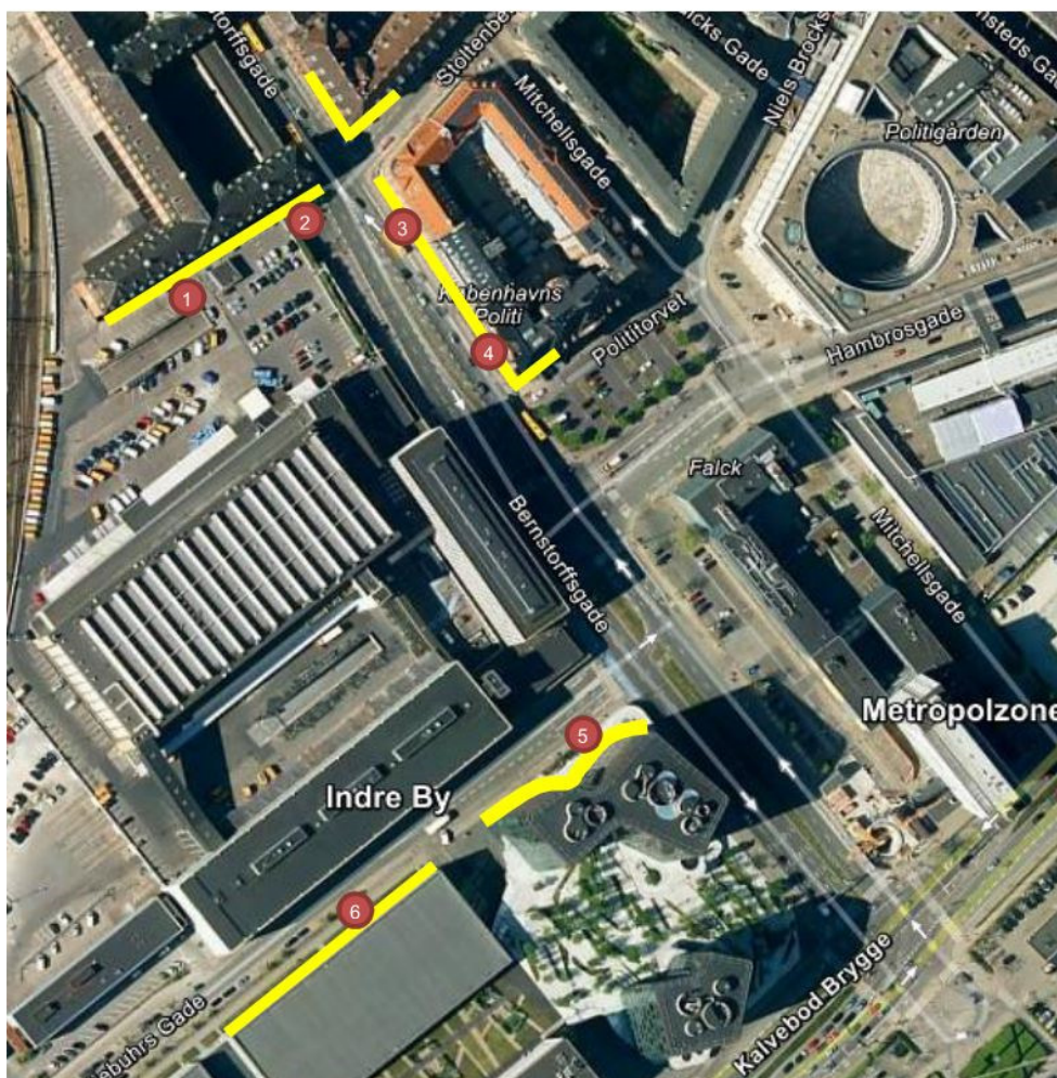
Billede 1, Placering af vibrationsmålere 1-6
